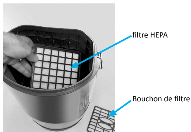
Figure 9 - Suppression de filtre HEPA
